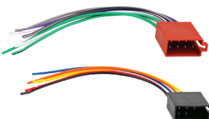
CONECTOR ISO MAMĂ
